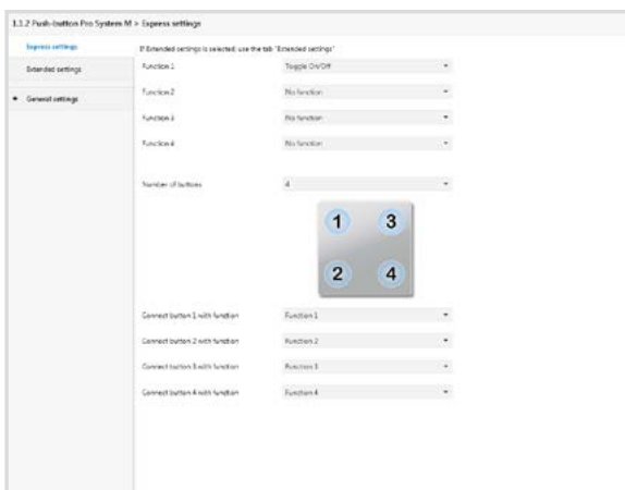
ETS gyorsbeállítások a KNX nyomó-vezérlő megoldásokhoz.
